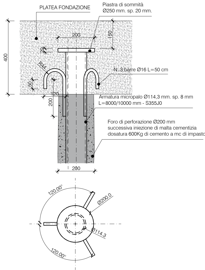
FONDAZIONI INDIRETTE - MICROPALI SCALA 1:10
